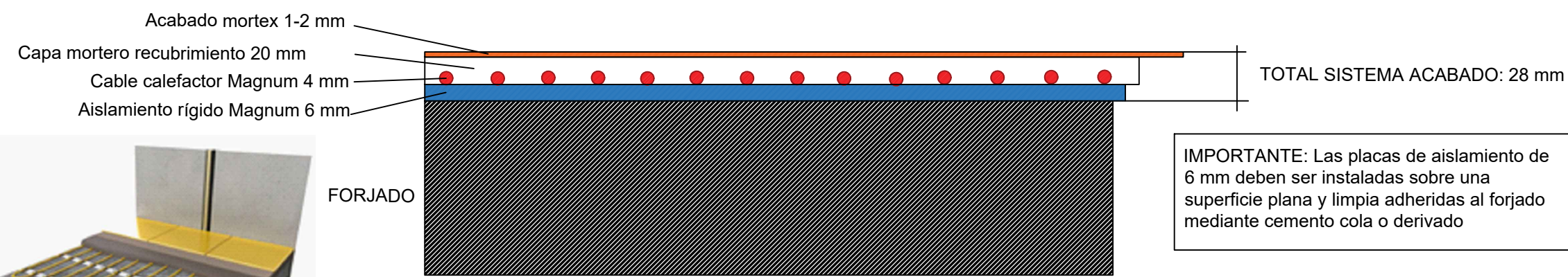
Sistema Cable MAGNUM con acabado Mortex
