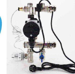
Sistema hidráulico
